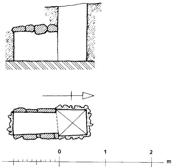
66. G 6014, shaft E: Elevation
