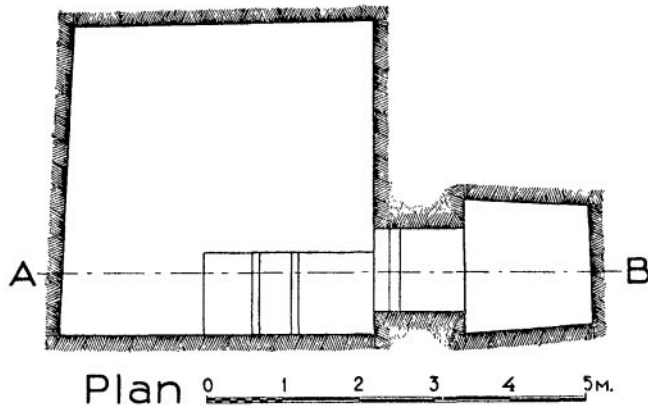
Plan 0 1 2 3 4 5 M. Fig. 292. G 4740
