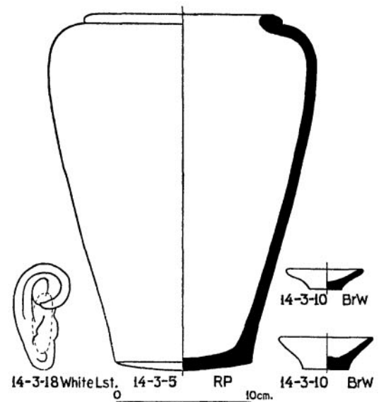
Fig. 325. G 4710
