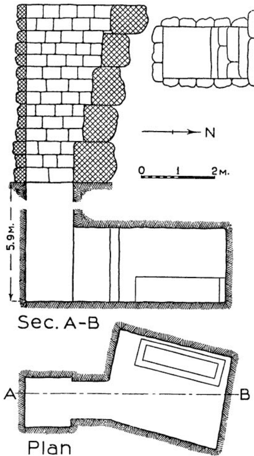
Fig. 319. G 4411 A
