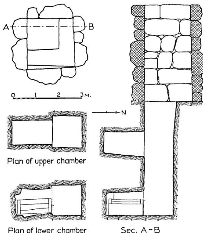
Fig. 316. G 4310 A
