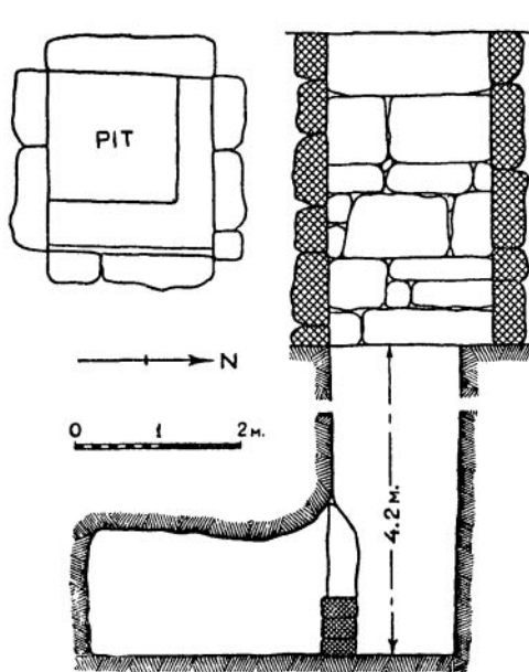
Section A-B
